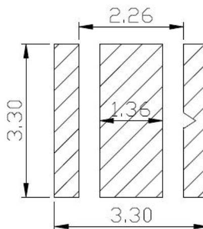
建议焊盘
